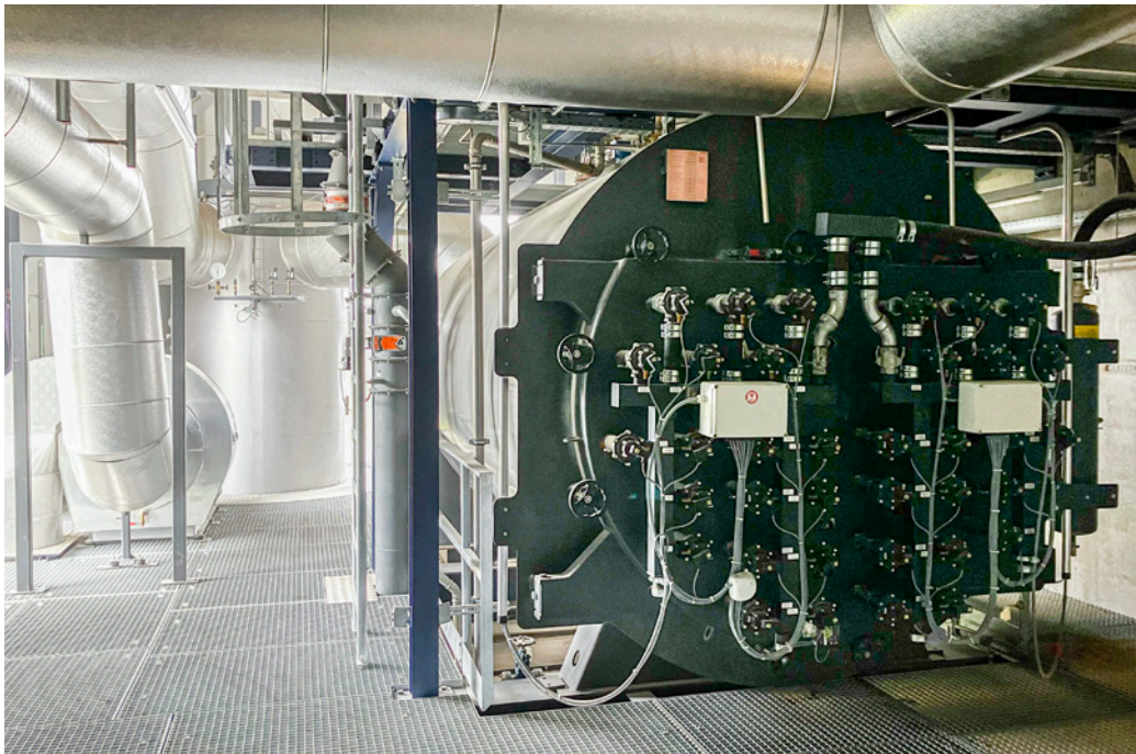
Heißwasseranlage
